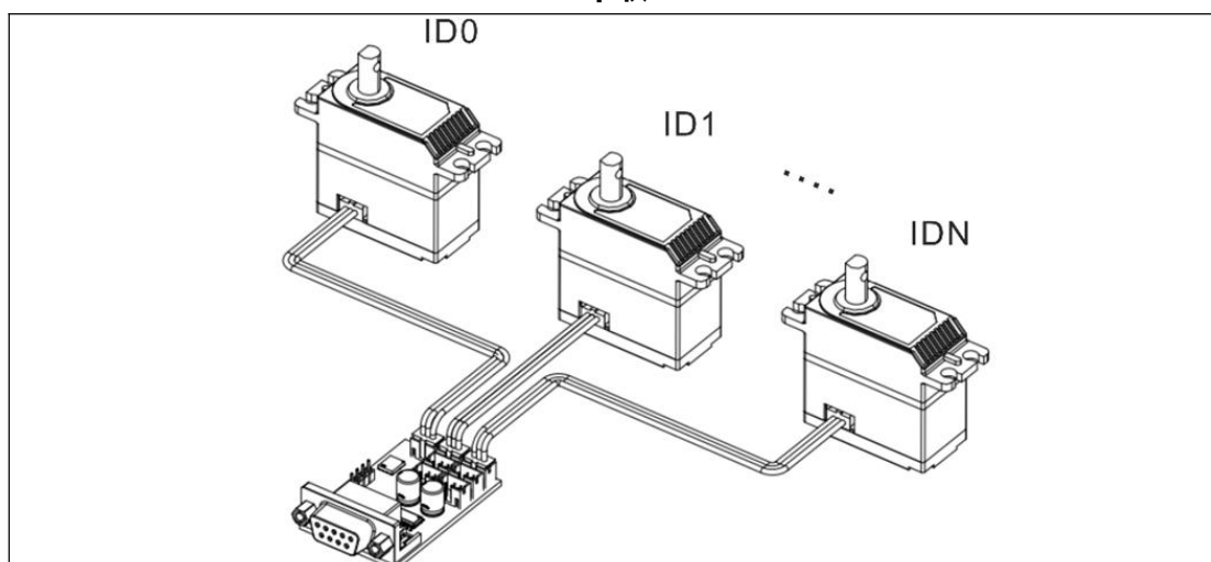
并联
