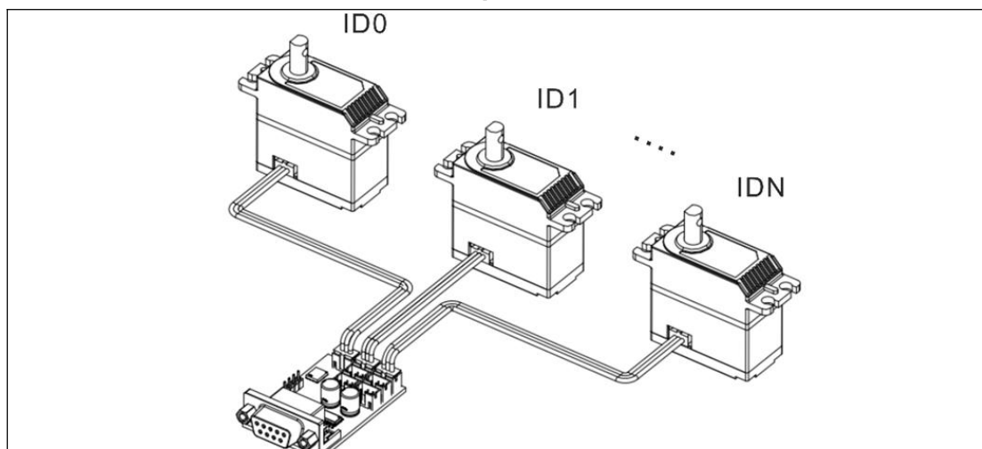
并联
