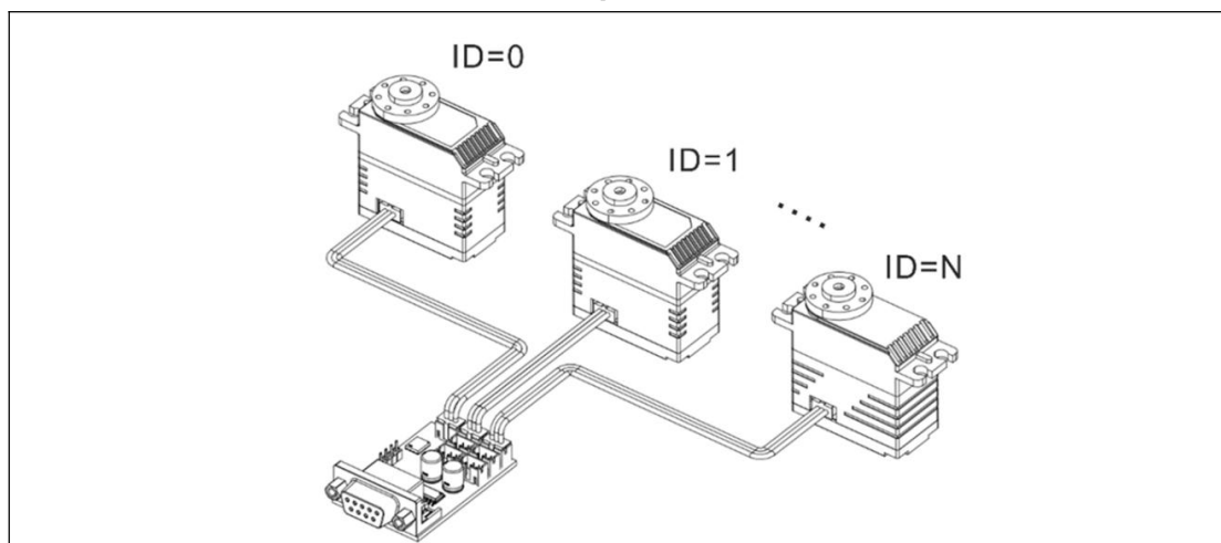
并联
